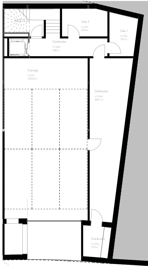
Planta Aparcamnet
