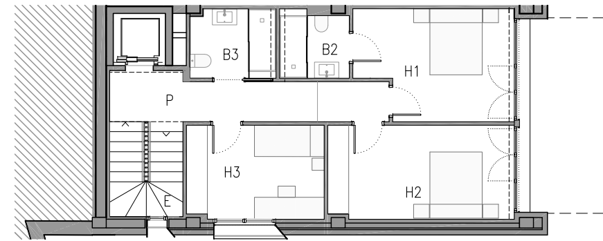
PLANTA PRIMERA
