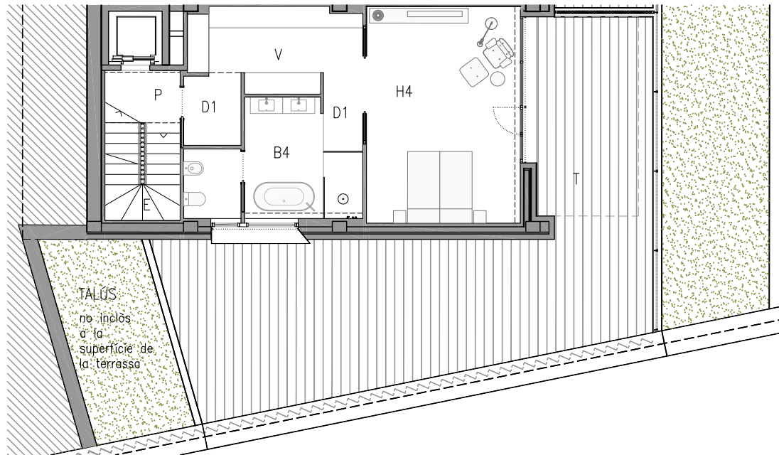
PLANTA BAIXA
